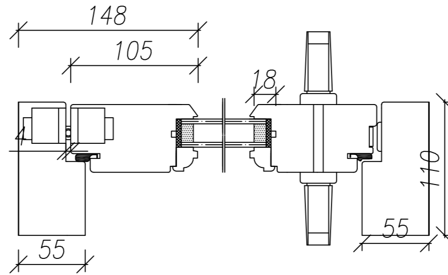
single door - hidden hinges
